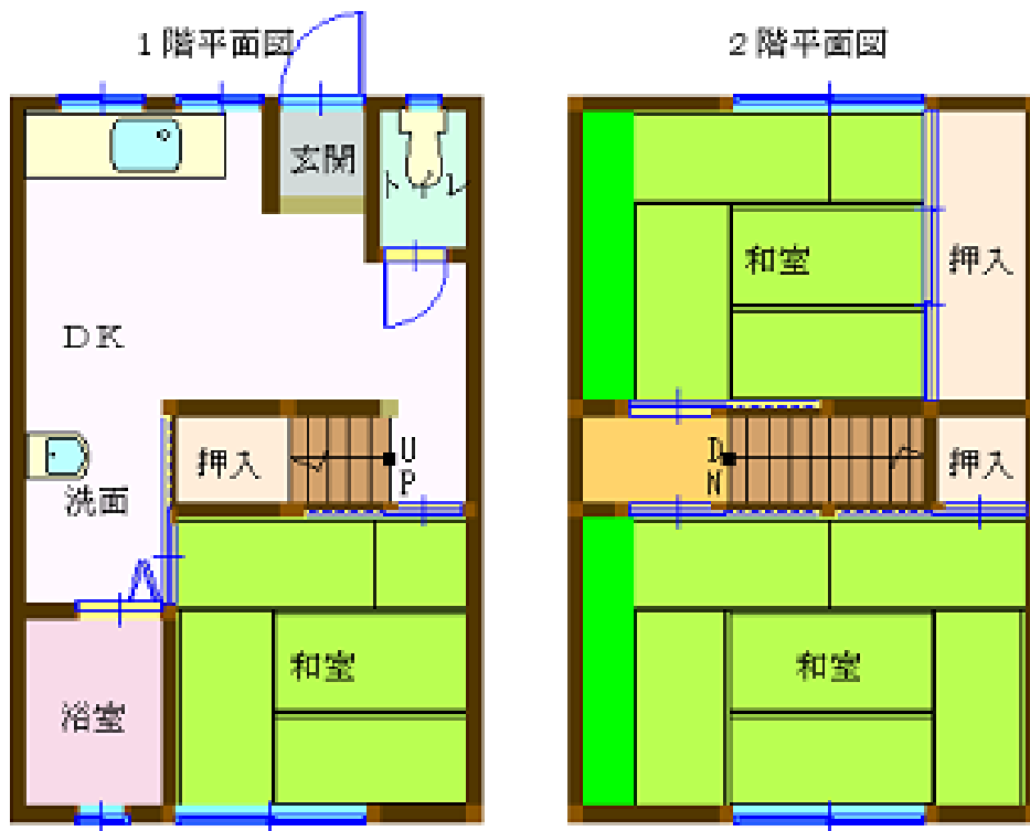
屋内見取り図
