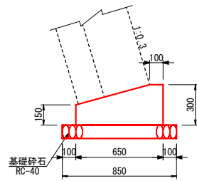
1号ブロック積基礎 S=1:20
