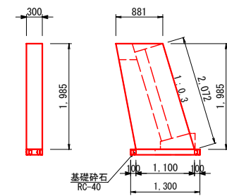
1号小口止コンクリート S=1:50
