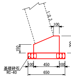
2号ブロック積基礎 S=1:20
