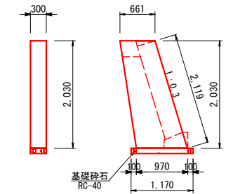
2号小口止コンクリート S=1:50
