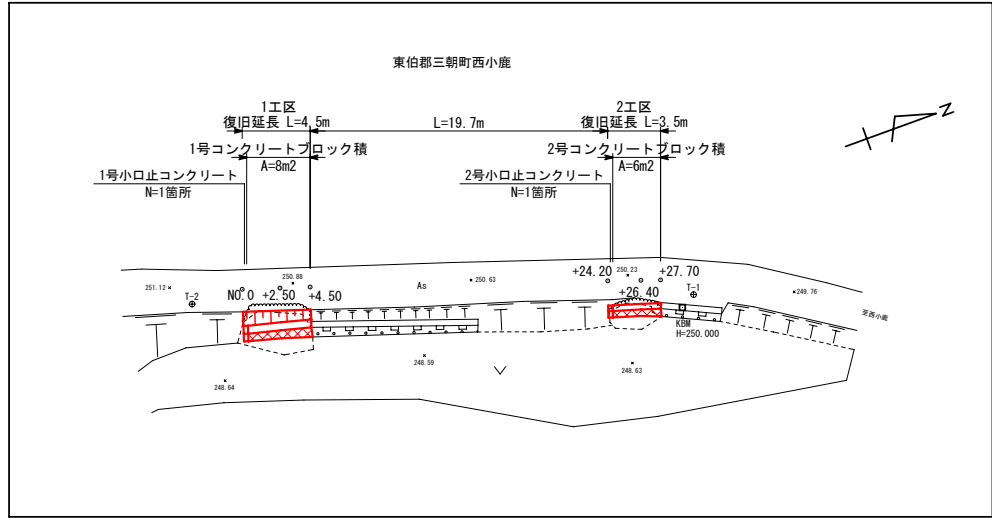
平面図 S=1:250
