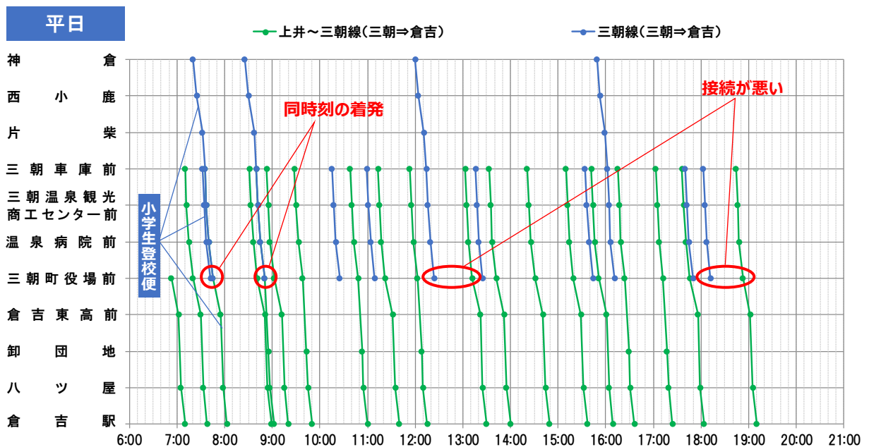
図 72 三朝線から上井・三朝線への乗換接続状況（上り）
