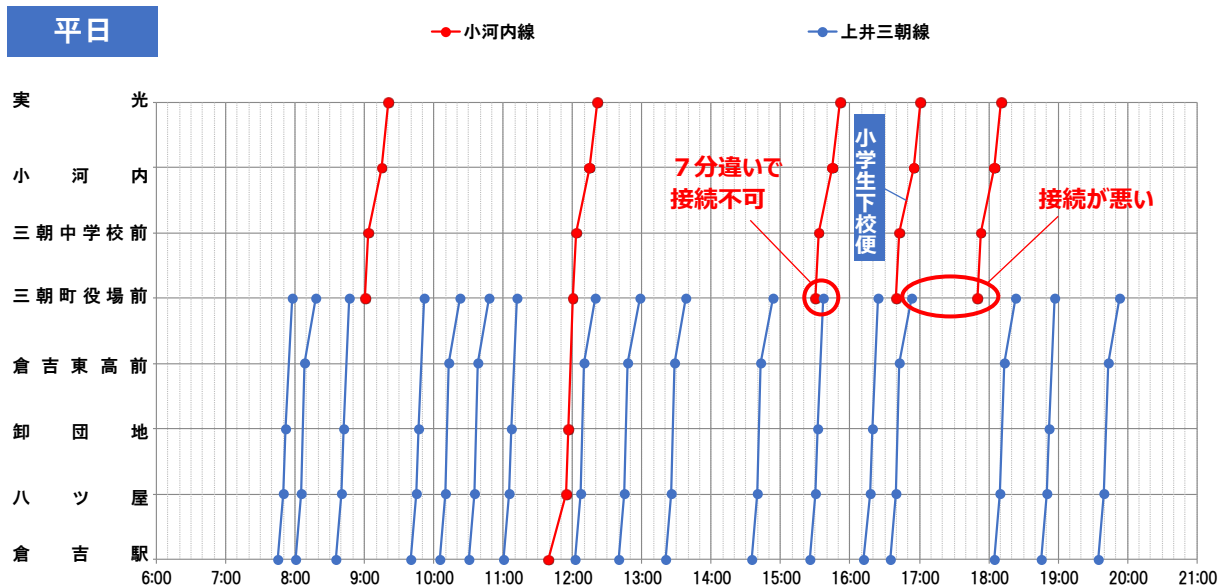
図 82 小河内線と上井・三朝線の接続状況（下り）
