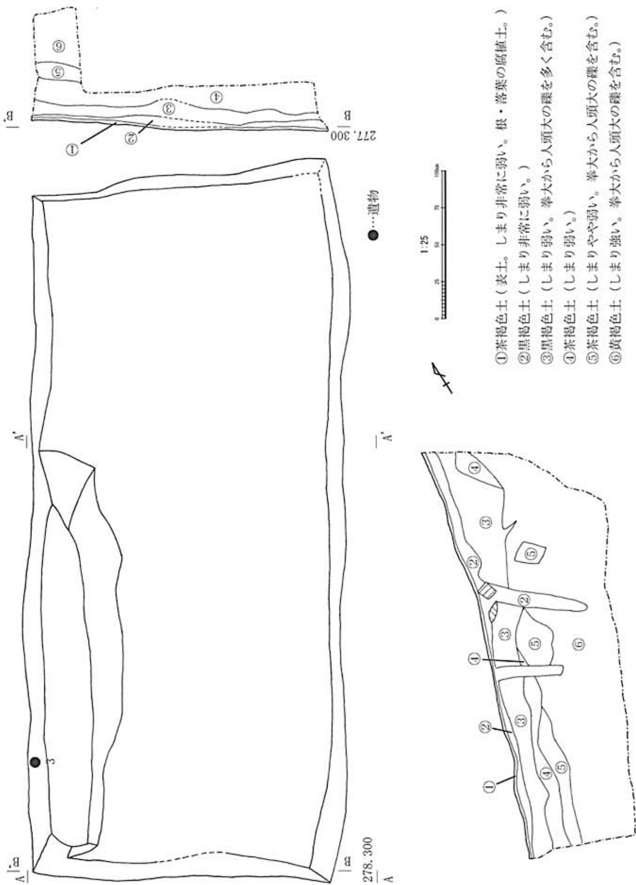
図8 第1地点 平面図・断面図
