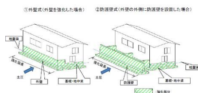
構造強化イメージ
