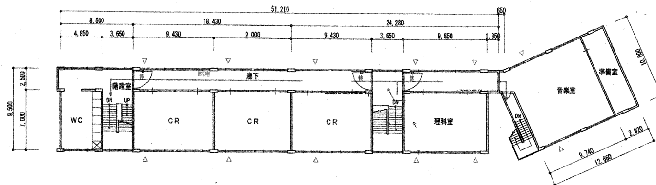
3階平面図 S=1:300
