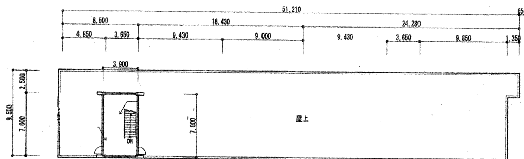
R階平面図 S=1:300
