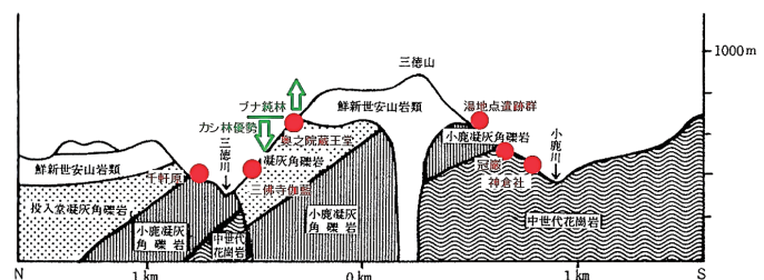
図6 三徳山の地質構造と植生・信仰遺跡の関係
