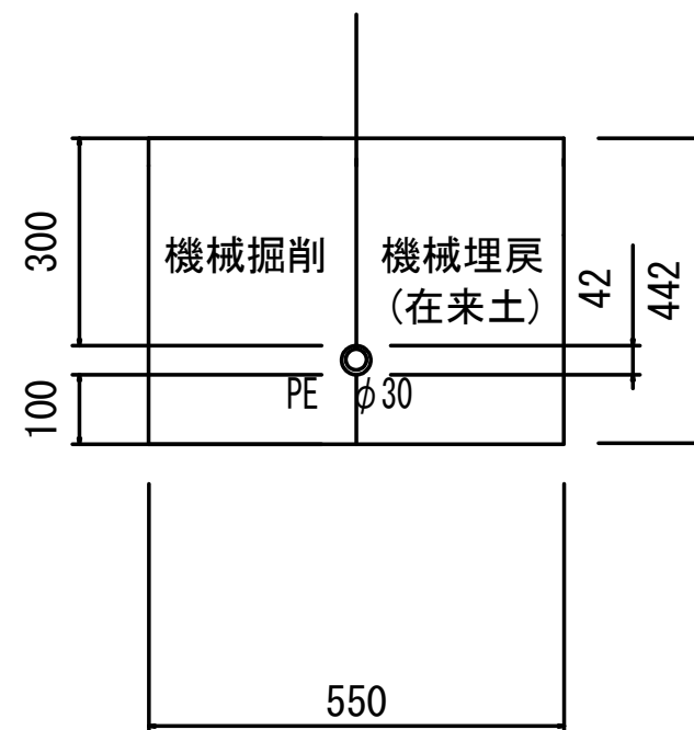
未舗装部断面図
