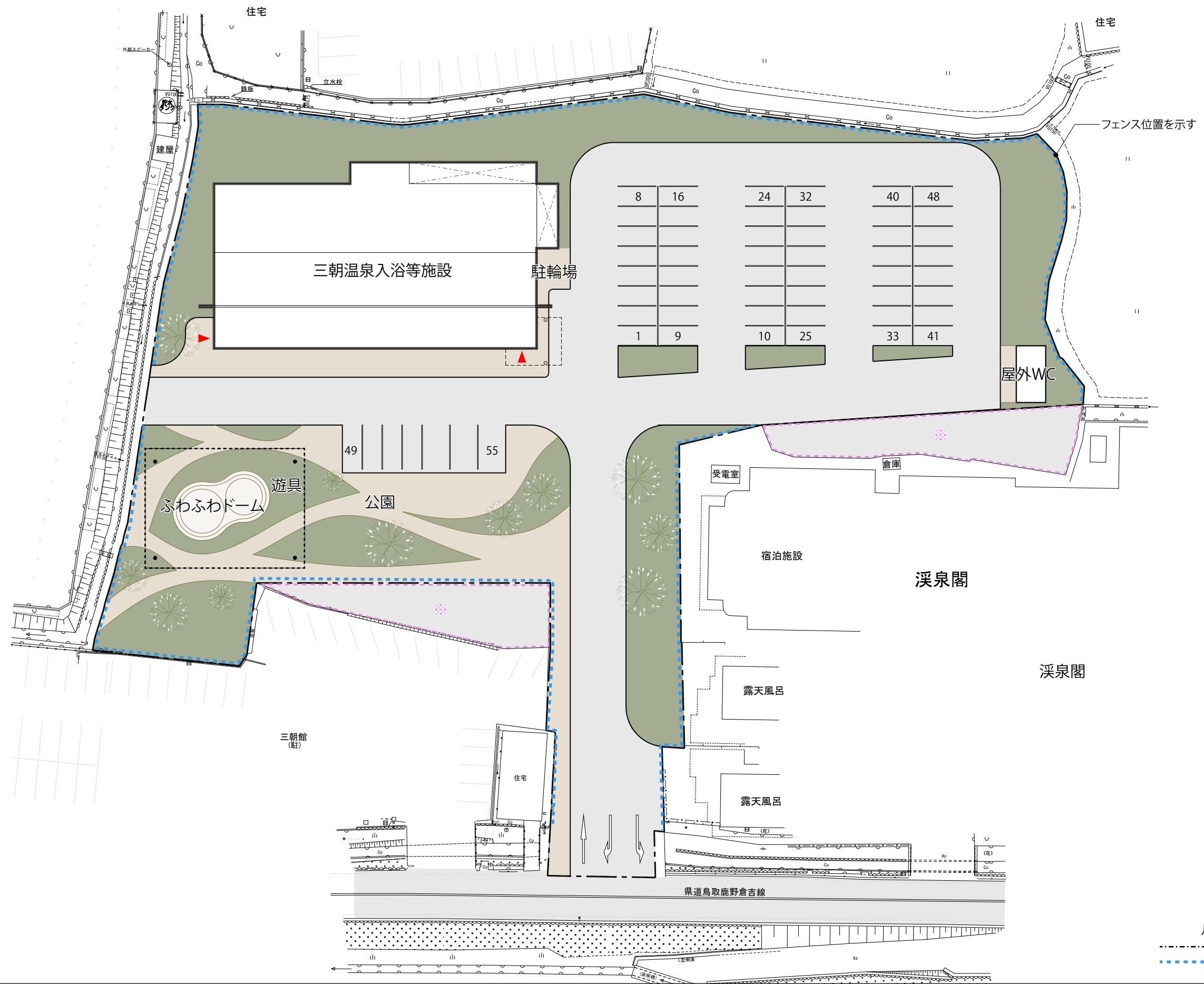
配置図
