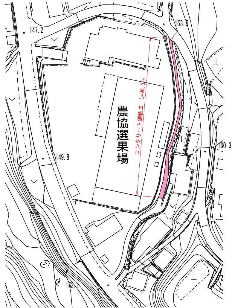
平面図 S=1:500
