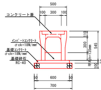
自由勾配側溝 (B300) S=1:20
