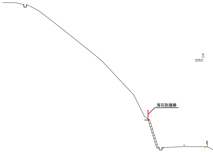
標準横断面図 1 : 100
