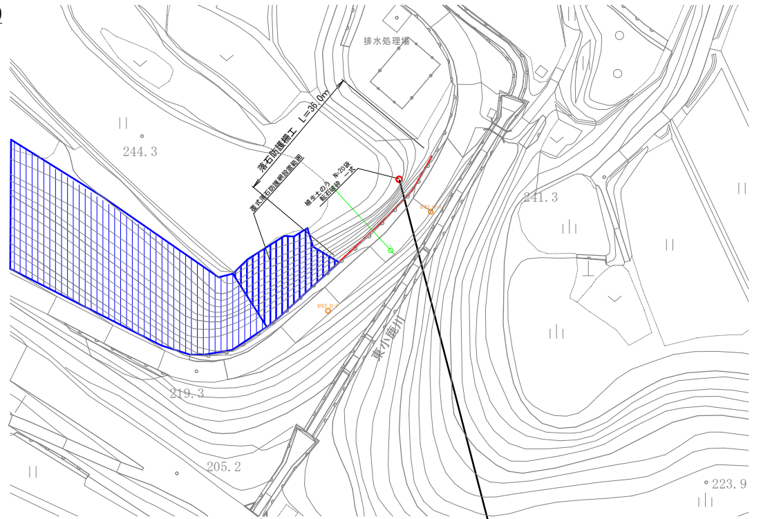
平面図 1 : 500
